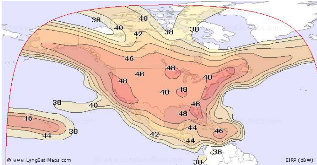
Empreinte des liaisons descendantes du Galaxy 19
