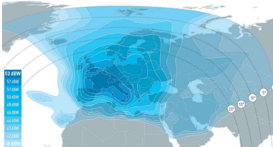
Empreinte des liaisons descendantes du Hotbird 13G
